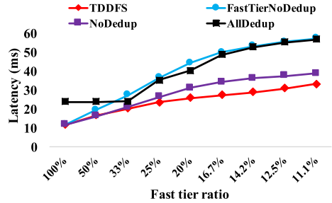
(d) Latency of Syn_trace
